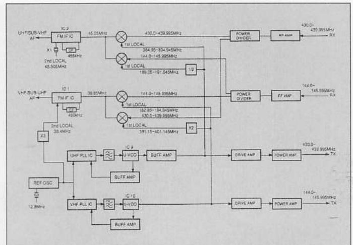
Figuur 2. Het blokschema van de opgewerkte frequenties.
